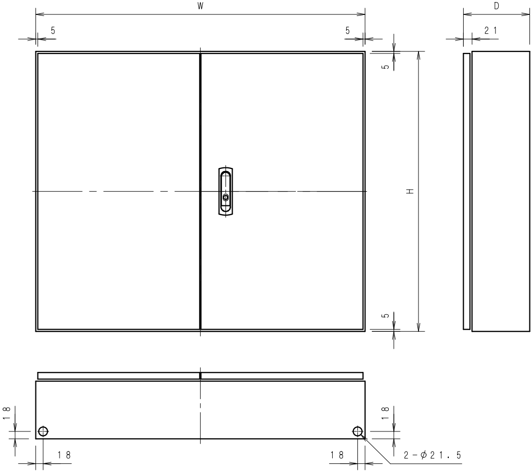
X P S Fシリーズ 両開き (W700~799)
