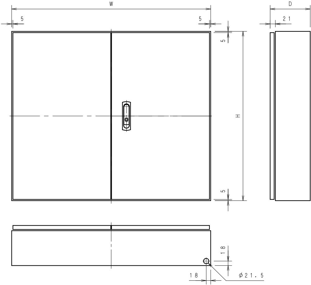
X P S Fシリーズ 両開き (W 6 0 0 ~ 6 9 9)
