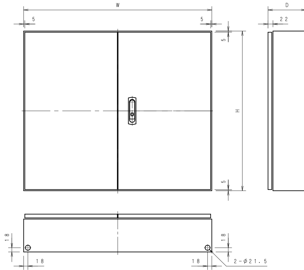
XATFシリーズ 両開き(W700~799)
