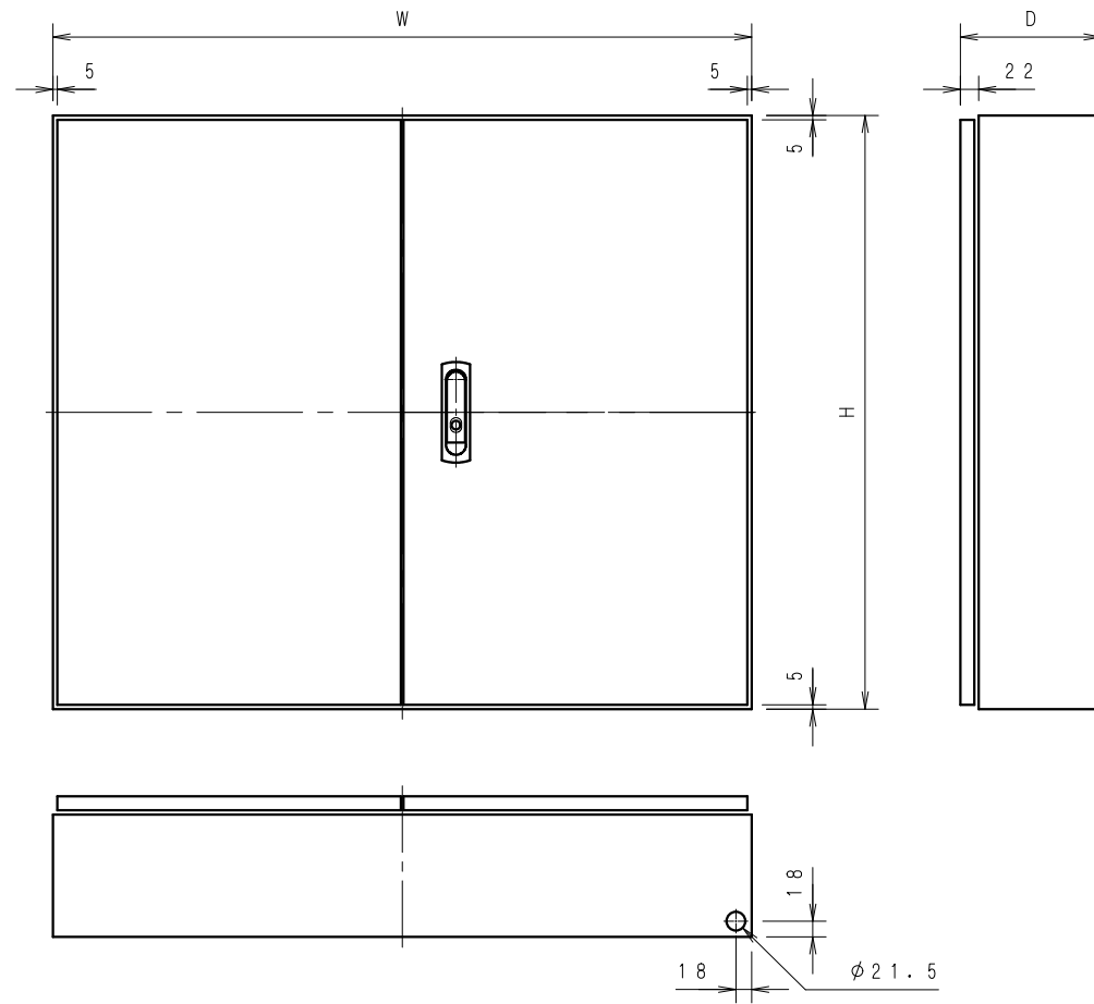
XATFシリーズ 両開き (W600~699)
