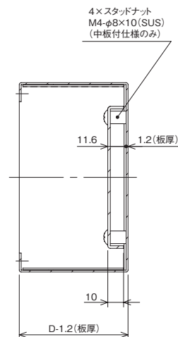
断面图 A-A
