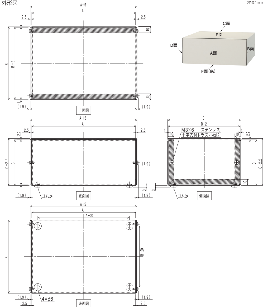
外形图
