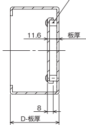
断面图 A-A
