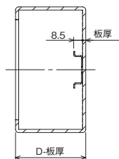
断面图 B-B
