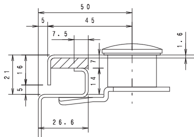
C部詳細
