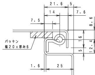
B部詳細
