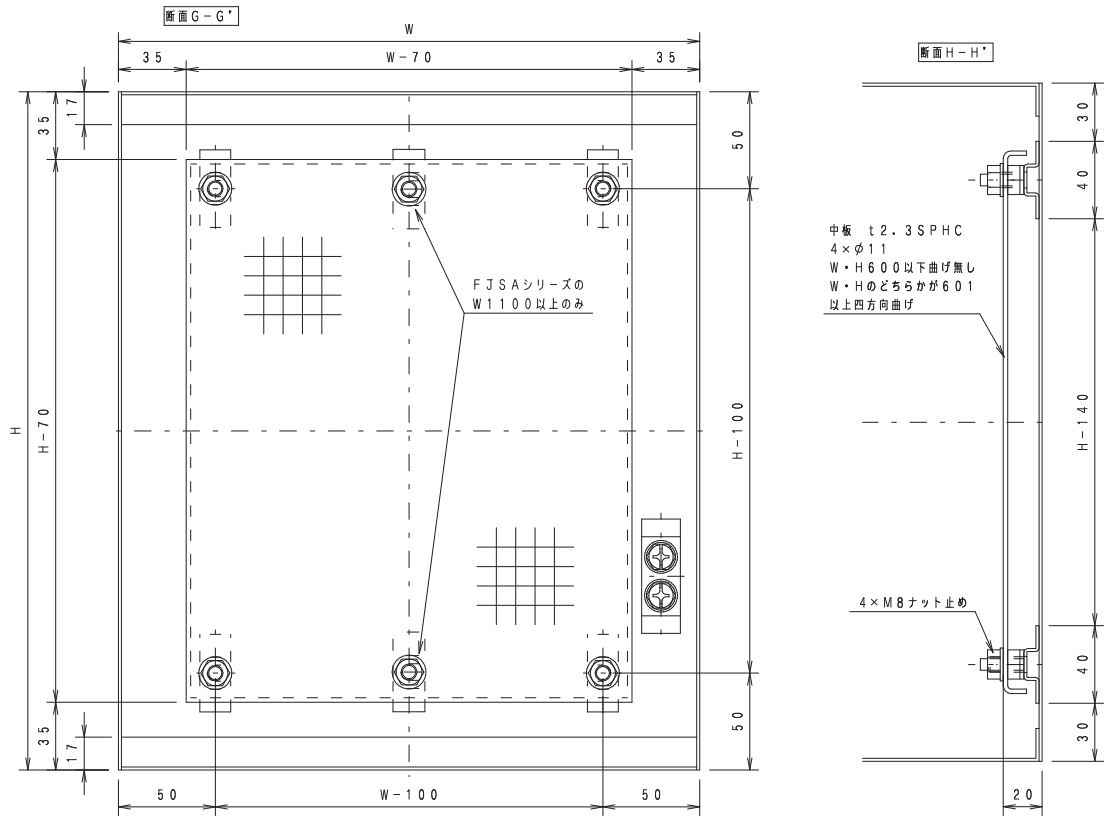
詳細図
