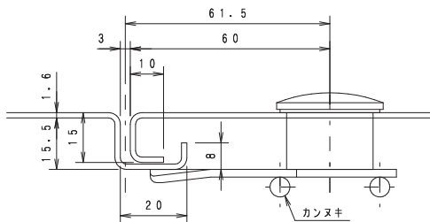
C部詳細
