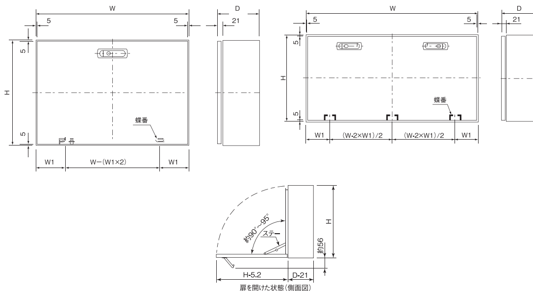
外形図
