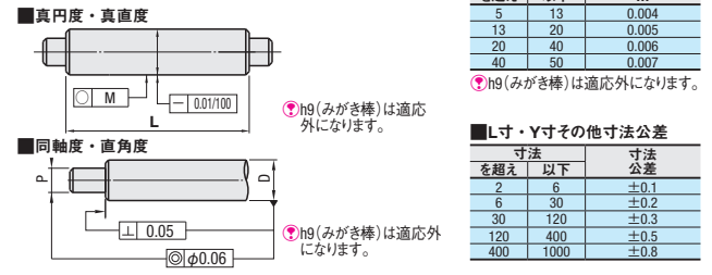
①D部公差h9(みがき棒)/P・Q部公差h7 ②D部公差h9(みがき棒)/P・Q部公差g6タイプ
