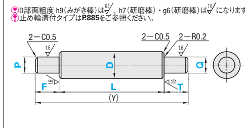
①D部公差h9(みがき棒)/P・Q部公差h7 ②D部公差h9(みがき棒)/P・Q部公差g6タイプ
