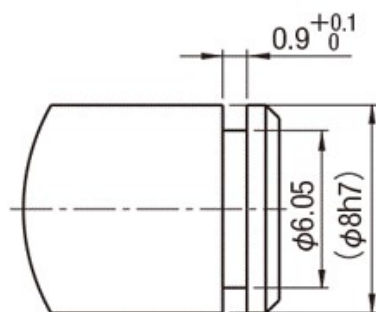
A詳細図
