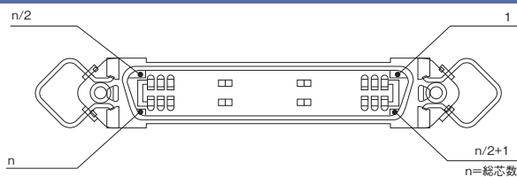
セントロニクスメスコネクタ コンタクト配列図
