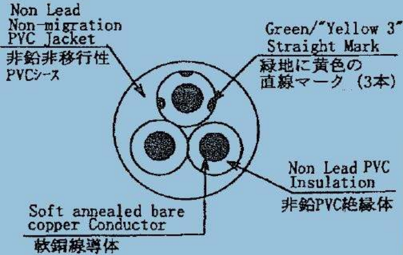
ケーブル断面
