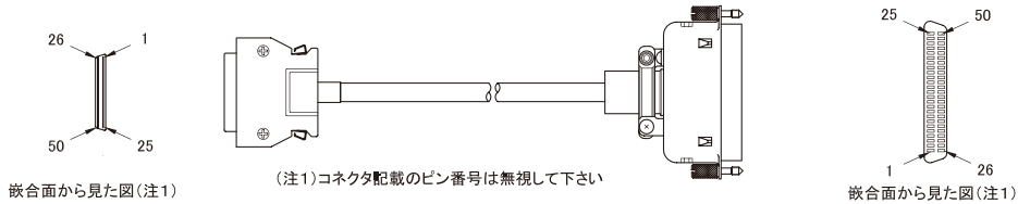
嵌合面から見た図(注1)
